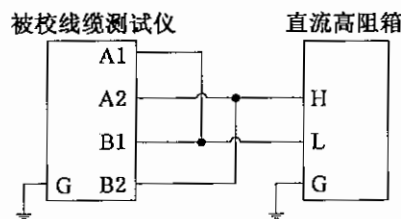
图 5 绝缘报警电阻校准接线图
