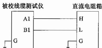
图 6 线缆直流电阻校准接线图
