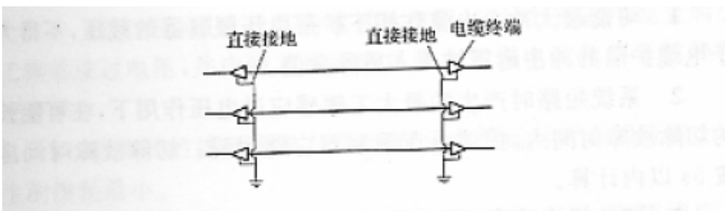
图 4.1.11-2 线路两端直接接地
