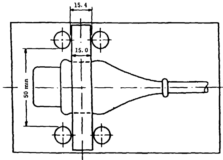
图 24 在连接器上进行压力试验的装置(见 24.1.3)
