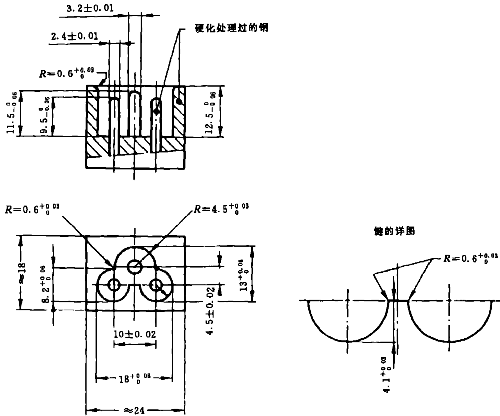
图 2 用于检查连接器是否符合图 C1 的通规(见 9.1)
