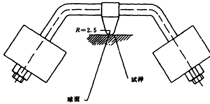
图 23 球压试验装置(见 24.1.2)
