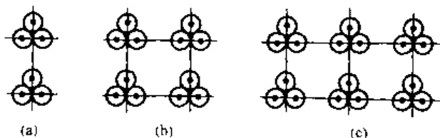
图 2-12-2 (a)、(b)、(c) 单芯典型的三角形
