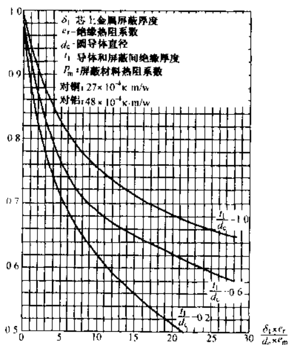
图 2-9-3 圆形三芯屏蔽电缆与相应无屏蔽电缆热阻之比
